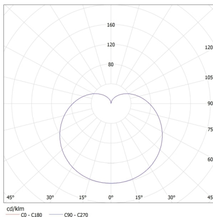
KANLUX S.A. (kat 23420) BILO 6,5W T SMD E27-WW / Krzywa rozsyłu światła (biegunowo)
