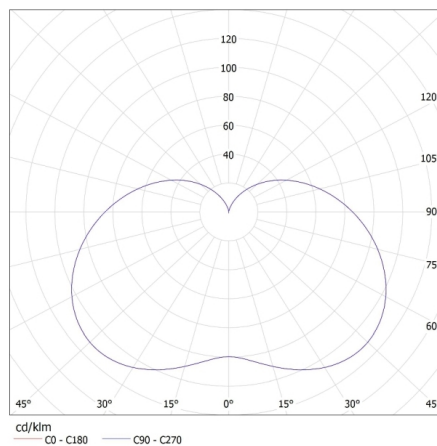
KANLUX S.A. (kat 23380) DUN 4,5W T SMD E14-WW / Krzywa rozsyłu światła (biegunowo)
