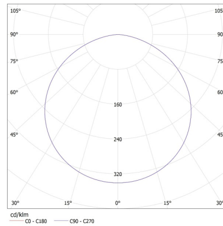
KANLUX S.A. (kat 24010) LEDS-P 4W/M IP00-WW / Krzywa rozsyłu światła (biegunowo)
